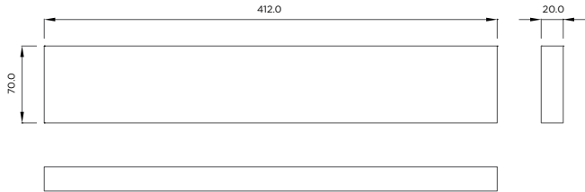
Letreiro Lona P vistas ortográficas
