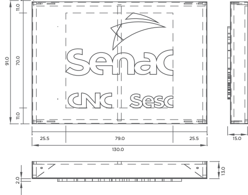
Totem Standard G vistas ortográficas do módulo da marca
