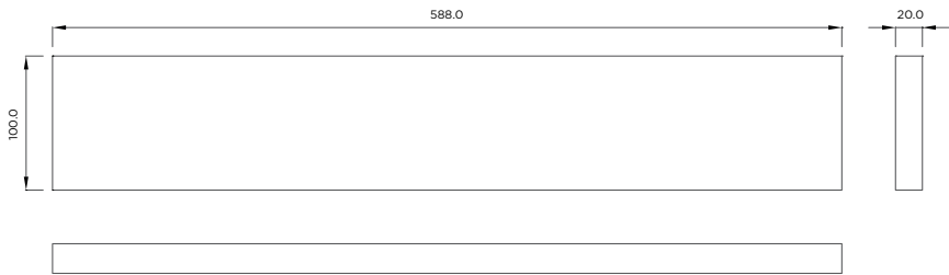
Letreiro Lona M vistas ortográficas
