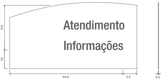
Chapa metálica vistas ortográficas do verso
