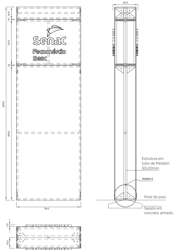
Totem Standard P vistas ortográficas gerais
