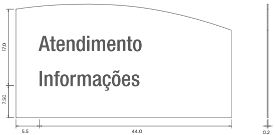
Chapa metálica vistas ortográficas da frente
