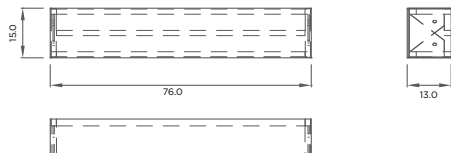
Totem Standard P vistas ortográficas do módulo reto superior
