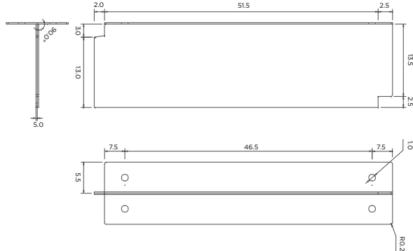
Chapa acrílica vistas ortográficas da frente
