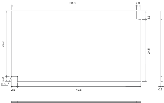
Chapa acrílica vistas ortográficas do verso
