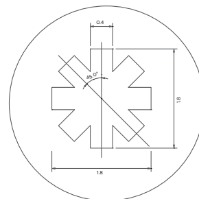
Detalhamento A
