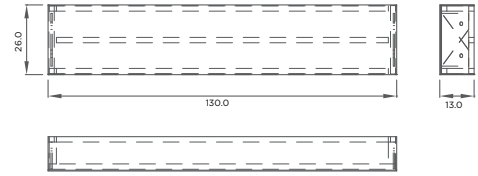
Totem Standard G vistas ortográficas do módulo da marca
