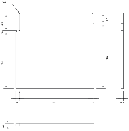
Chapa acrílica vistas ortográficas
