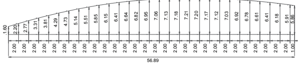
Chapa metálica flecha
