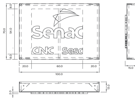
Totem Standard M vistas ortográficas do módulo da marca
