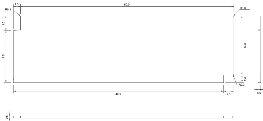
Chapa acrílica vistas ortográficas
