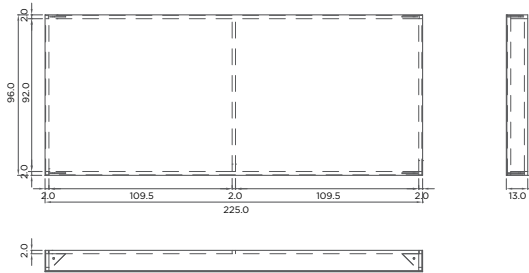
Letreiro Standard G2 vistas ortográficas do módulo reto
