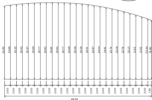
Chapa metálica flecha
