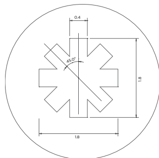
Detalhamento A
