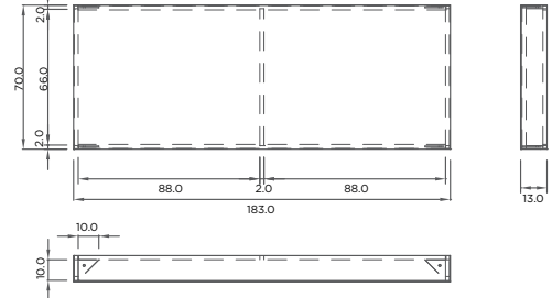
Letreiro Premium P vistas ortográficas do módulo convexo
