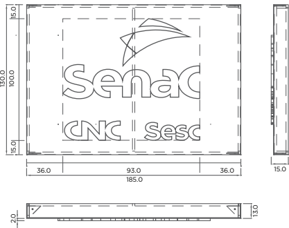
Letreiro Standard G2 vistas ortográficas do módulo da marca
