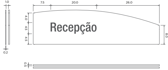
Chapa metálica vistas ortográficas da frente
