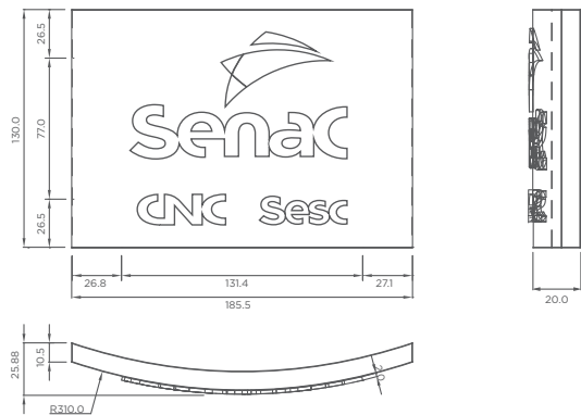
Letreiro Premium G vistas ortográficas do módulo da marca
