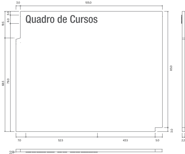
Chapa acrílica vistas ortográficas
