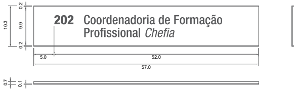
Chapa metálica régua dupla
