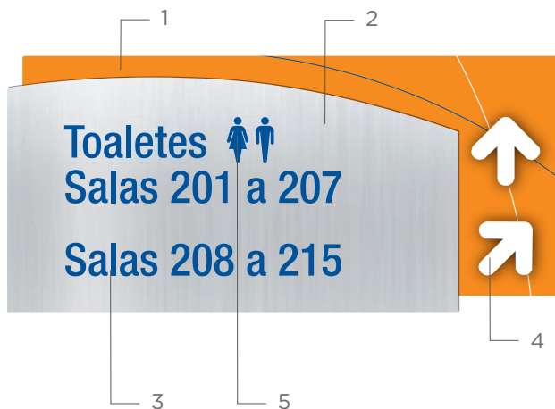
Detalhamento fixação
