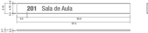
Chapa metálica régua simples
