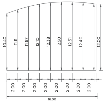
Chapa metálica flecha
