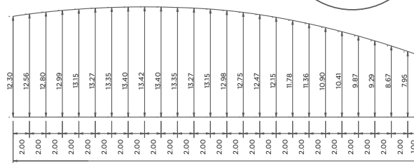
Chapa metálica flecha
