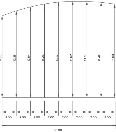
Chapa metálica flecha
