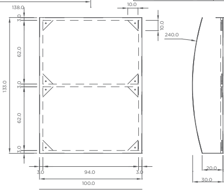
Totem Premium G vistas ortográficas do módulo convexo
